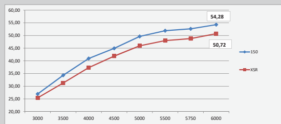
MAKSIMALNA POTROŠNJA GORIVA (l/h)
