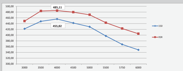
OKRETNI MOMENAT NA OSOVINI ELISE (Nm)
